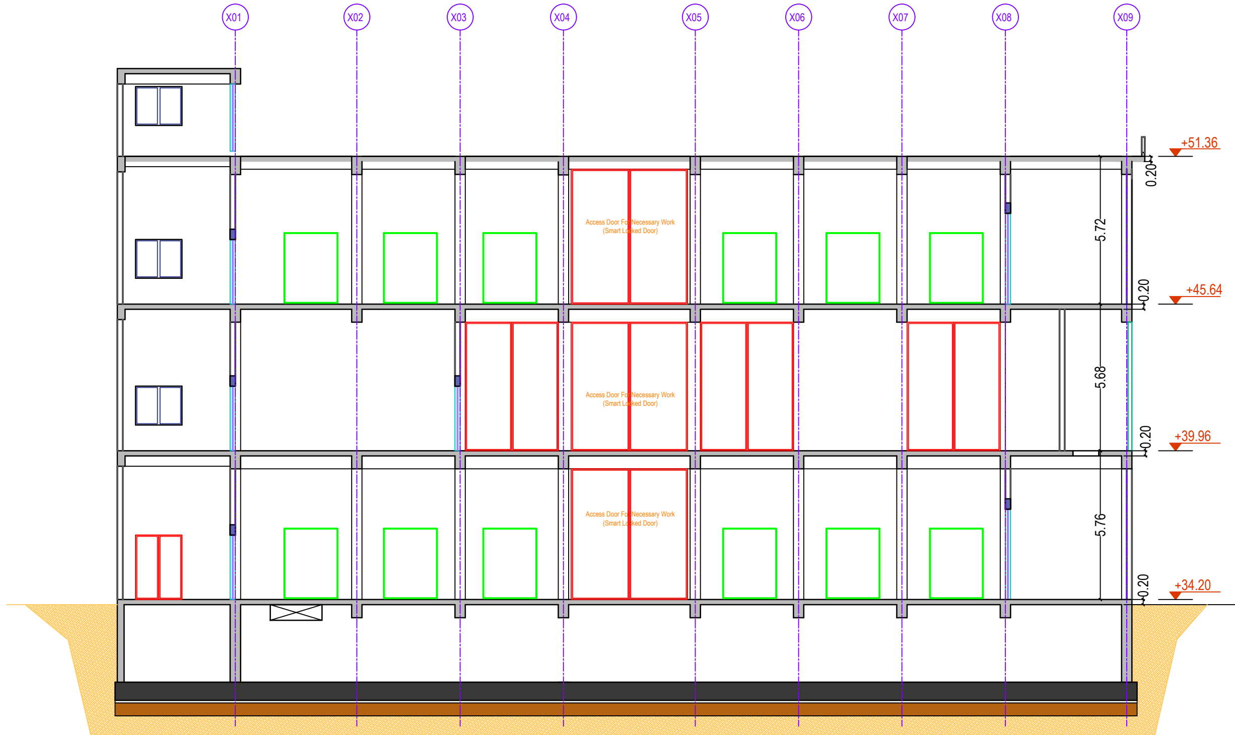
Section A-A
