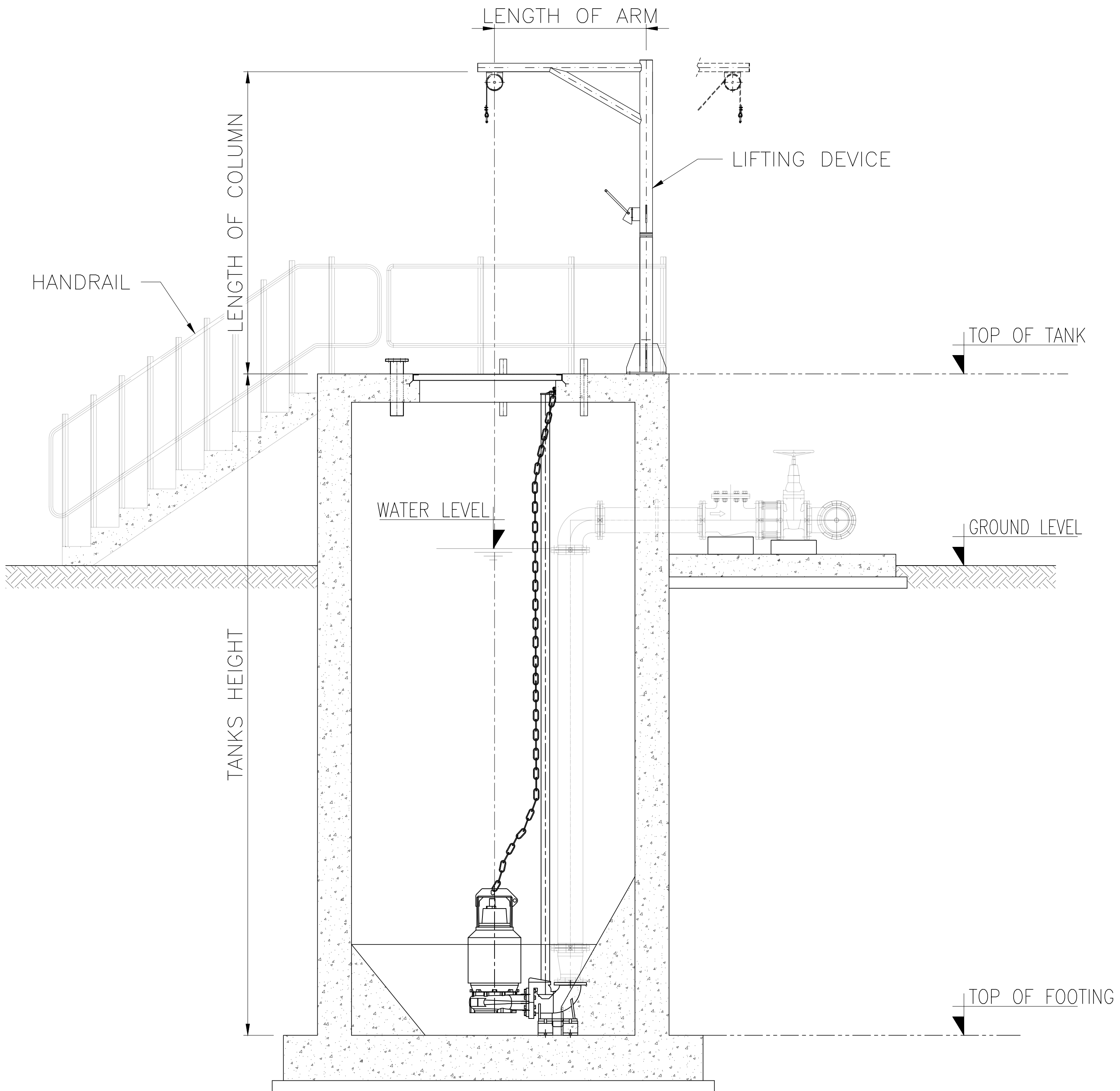
SECTION SCALE N.T.S
